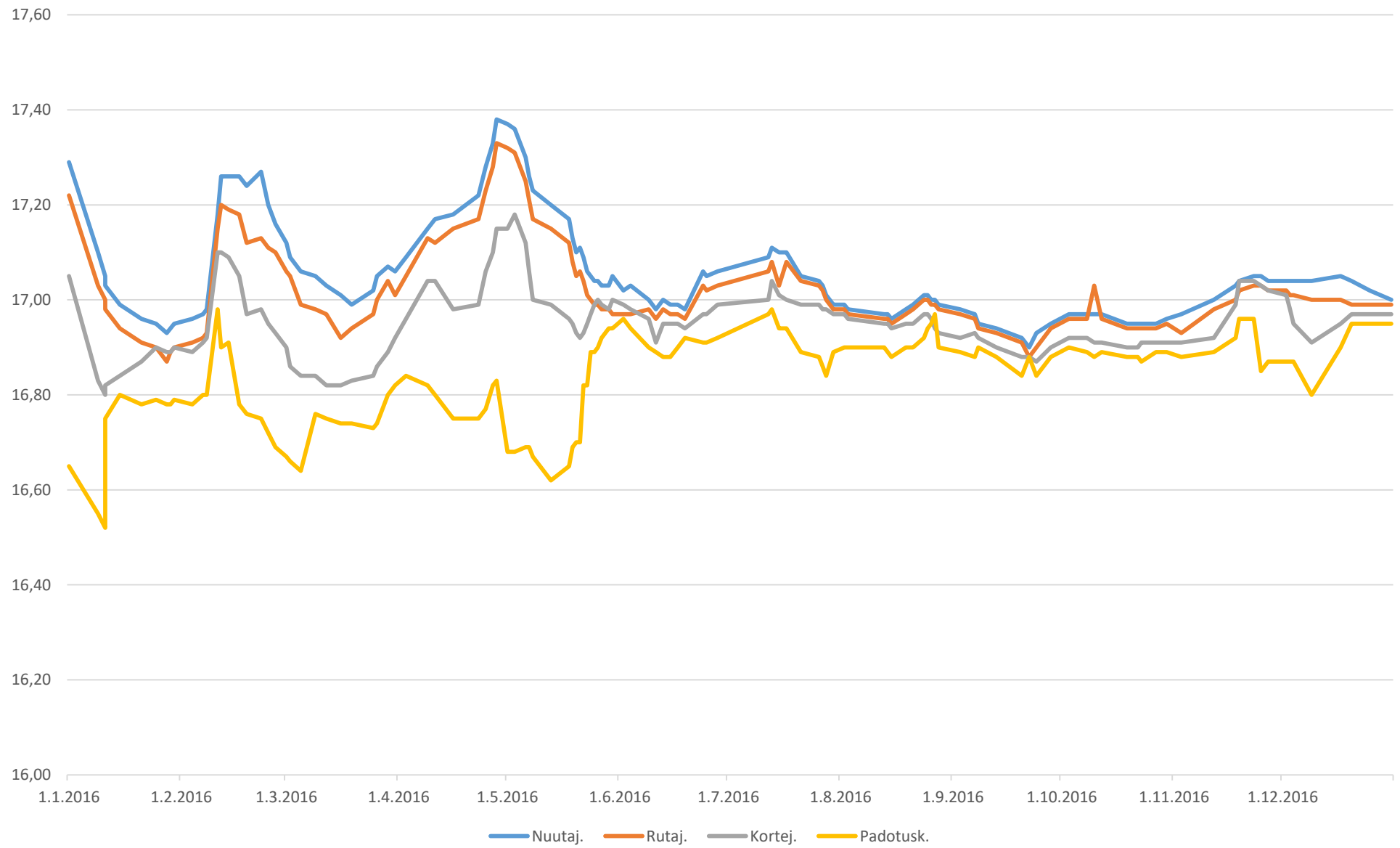
Nuutajärven, Rutajärven ja Kortejärven vedenkorkeudet sekä padotuskorkeus v. 2016
